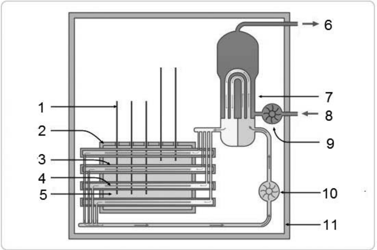
రియాక్టర్ను చల్లబరిచి ఆవిరిని తయారుచేసే ప్రక్రియ
